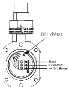
Figure 4: Connexions de câble sur site sur l' IRmax
