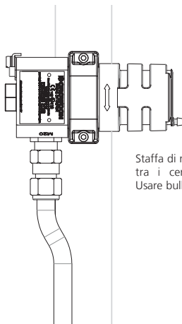
Schema 5: rilevatore IRmax con staffa di montaggio e pressacavo
