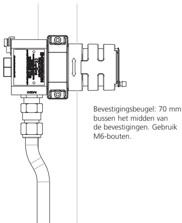
Afbeelding 5: De IRmax detector met een montagebeugel en kabelpakking
