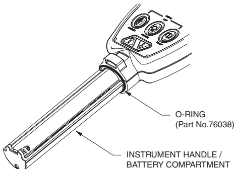
Fig. 13.12 Replace O-Ring
